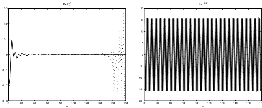
Fig. 10 - Example 1: Values for \text{Re } l_j^{(n)} , \text{Im } l_j^{(n)} .
