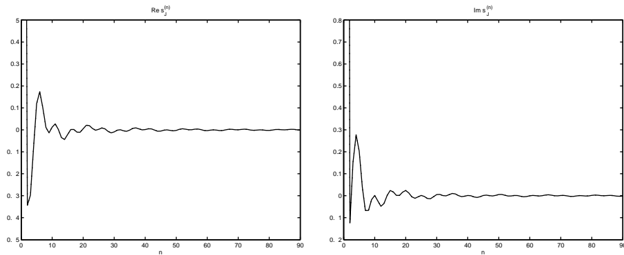
Fig. 11 - Example 1: Values for \text{Re } s_j^{(n)} , \text{Im } s_j^{(n)} .
